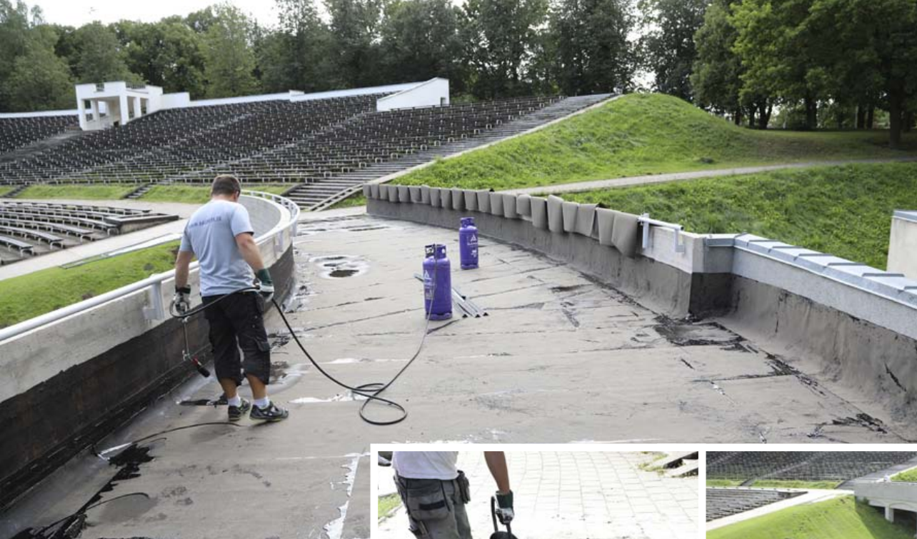
Kuumliimitav bituumenrullmaterjal paigaldatuna
